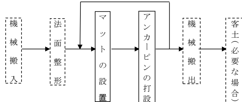
図2-1 施工フロー
