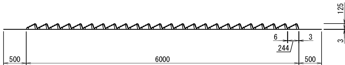
側面図 S=1:50
