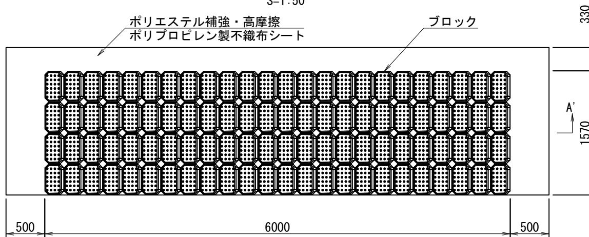
平面図 S=1:50
