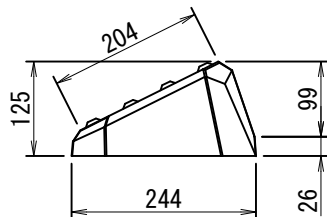
側面図 S=1:10
