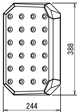
平面図 S=1:10
