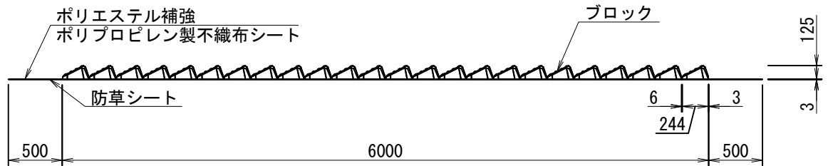
側面図 S=1:50
