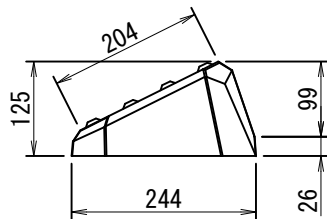
側面図 S=1:10
