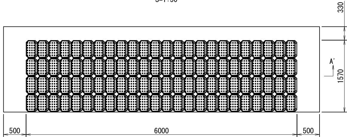
平面図 S=1:50
