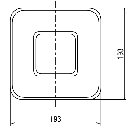
平面図 S=1:5
