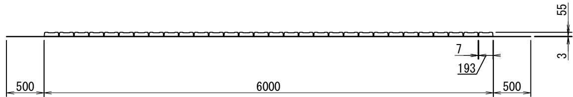
側面図 S=1:50
