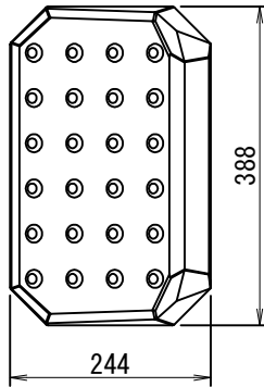
側面図 S=1:10
