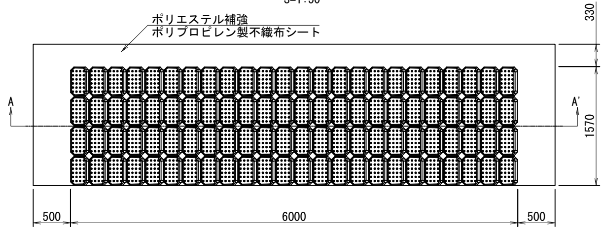
平面図 S=1:50
