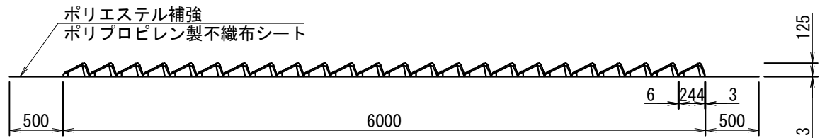
A-A' 断面図 S=1:50
