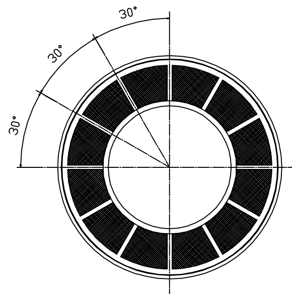
A-A' 矢視図
