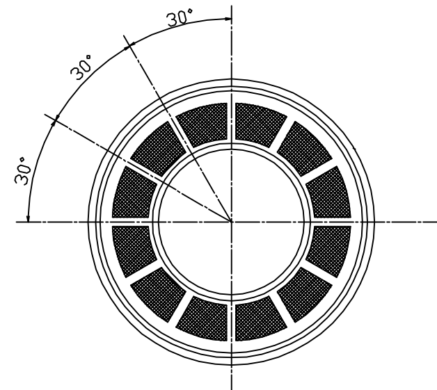
A-A' 矢視図
