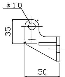
右側面図
