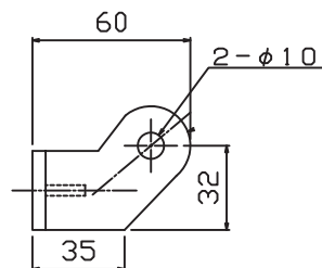
右側面図
