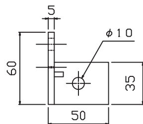
正面図
